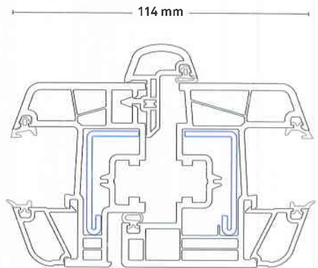
Arcade klassisch Stulpausführung Abb.: 1:2
